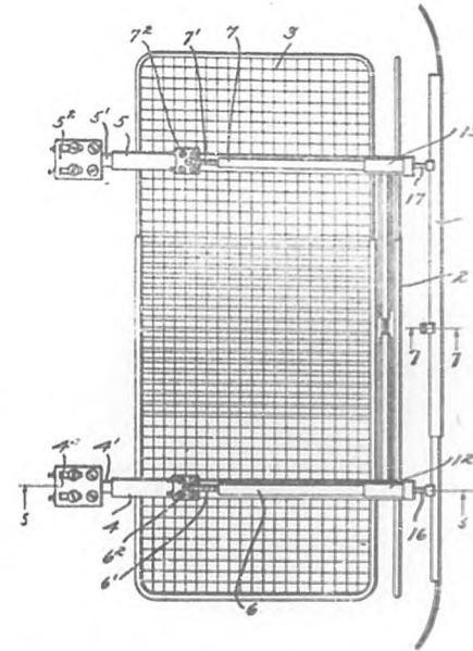
DEFENSA AUTOMATICA PARA VEHICULOS. —Cuadrangular de alambre enrejado que baja hasta el nivel del pavimento.
